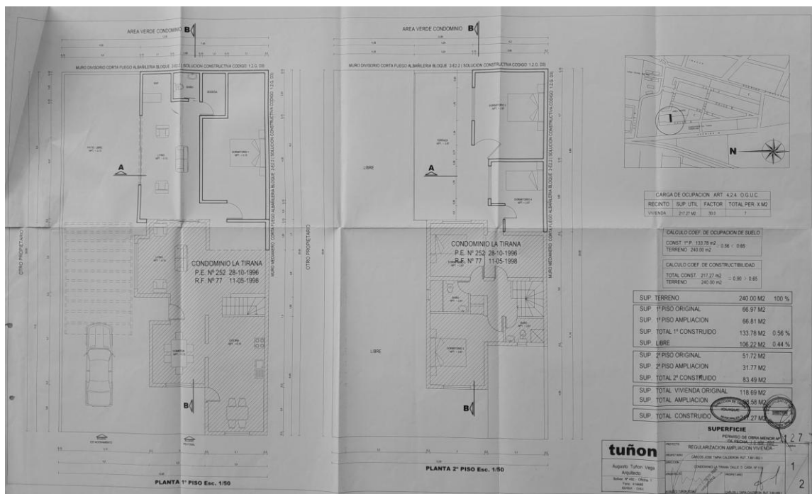
PLANO AMPLIACIÓN 2013
